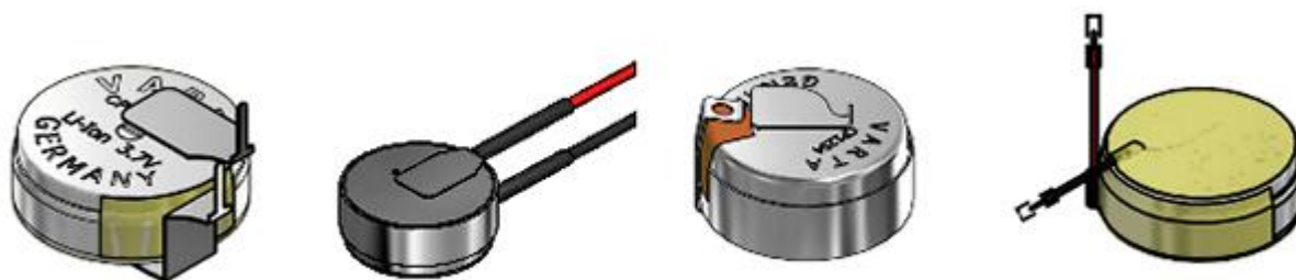
Рис. 11. Форма выводов аккумулятора.
