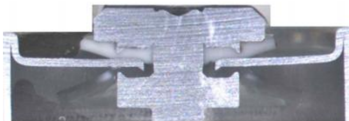
Рис. 3. Конструкция LiSOCl 2 батареи VARTA
